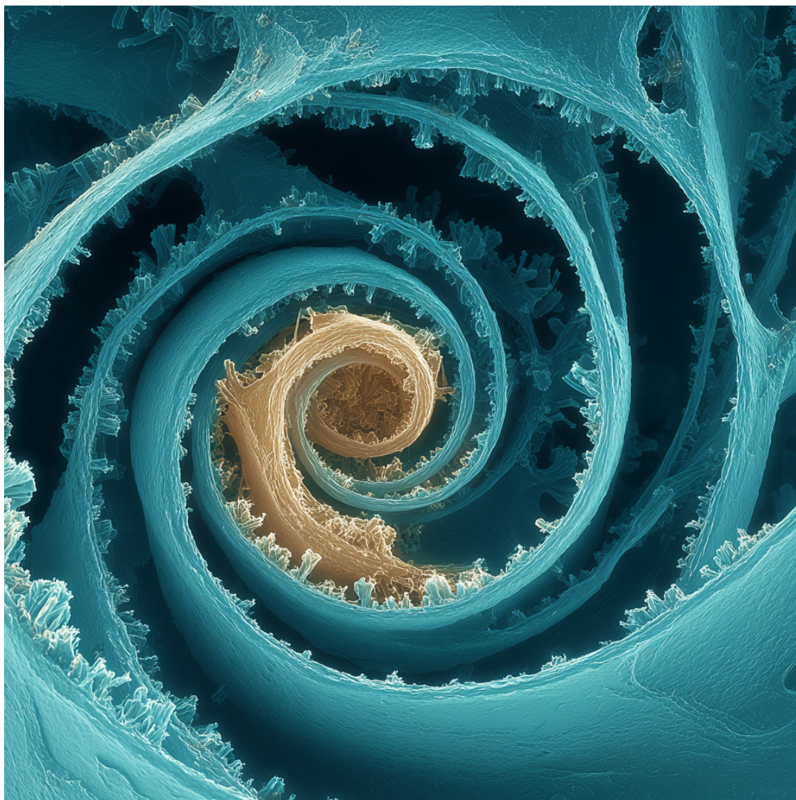
Figura 8: [\Psi \cdot \text{OBS}] L20-EM-spirale-mdes008-007
